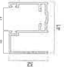
Guida in alluminio GJIAL32x41 DISTANZIALE
